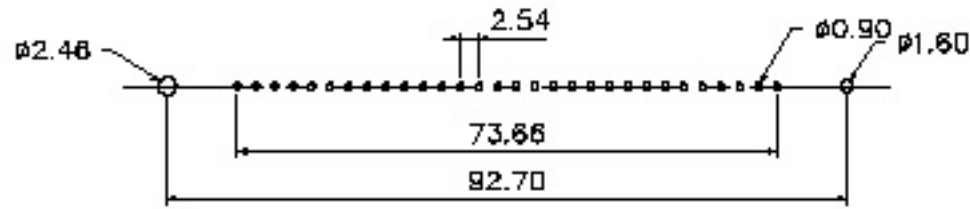
P.C.B. Layout
